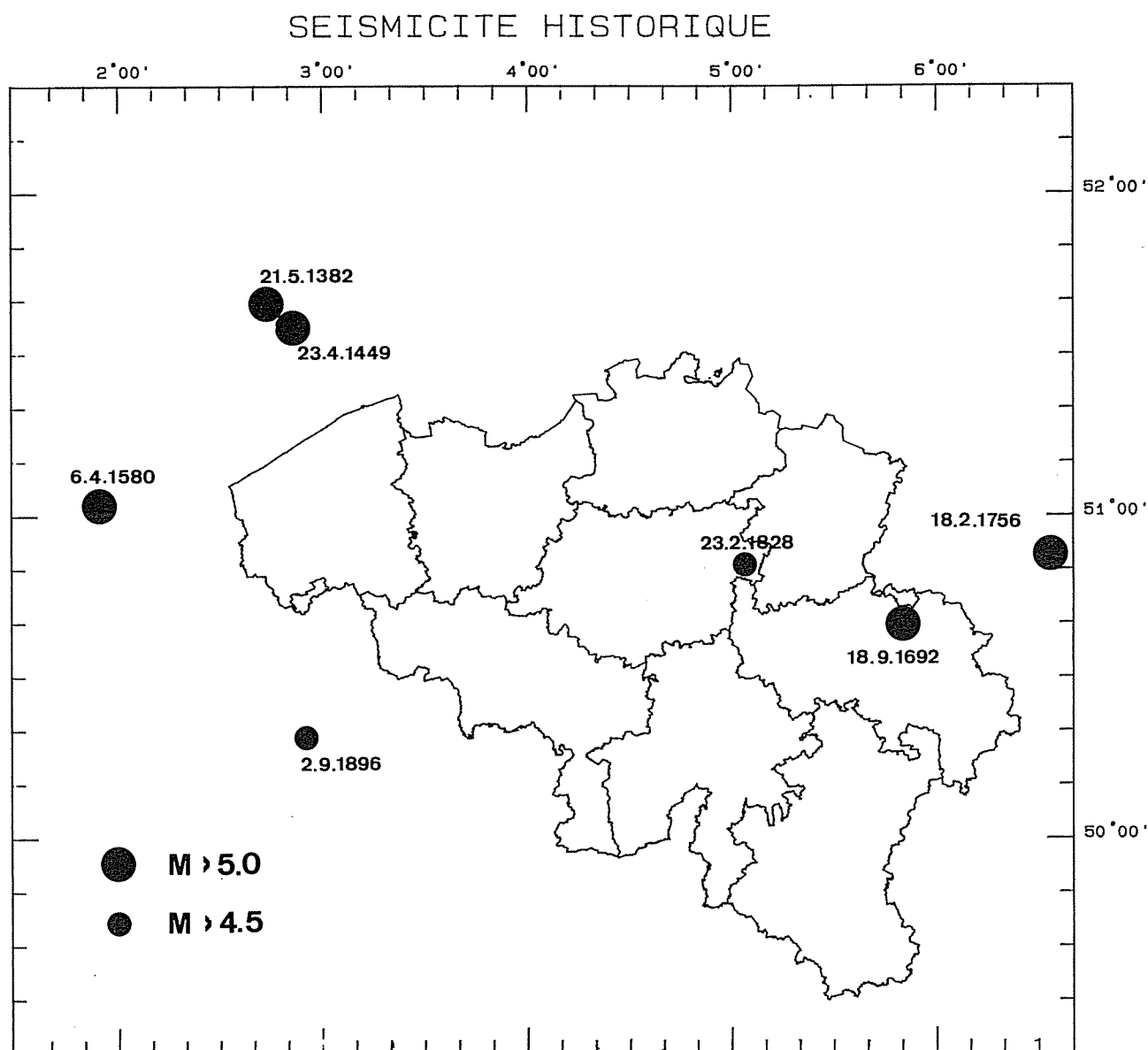
Fig. 5.- Localisation des séismes historiques importants ressentis en Belgique (avant 1910).
