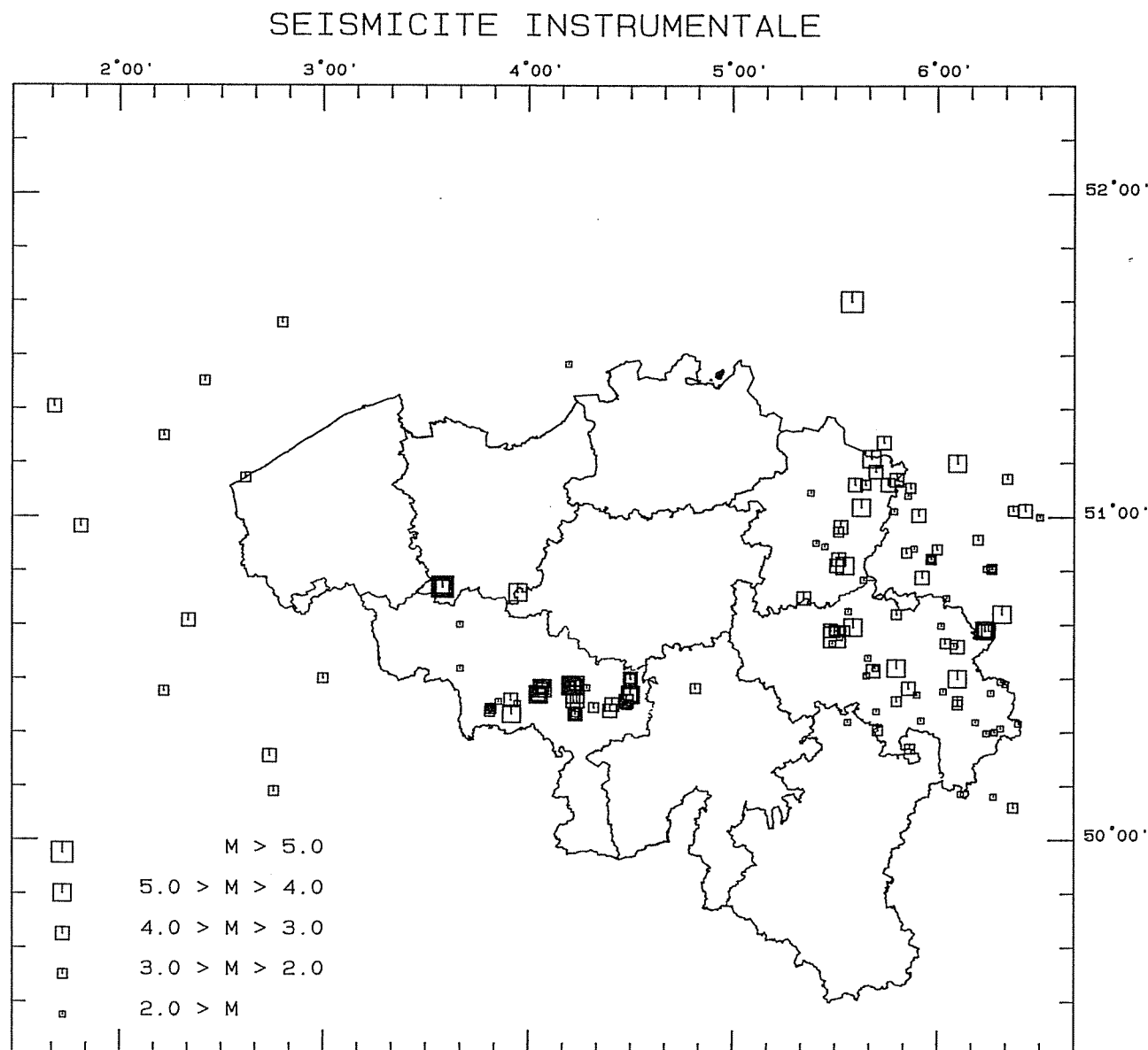
Fig. 4.- Séismicité instrumentale en Belgique (depuis 1910).
