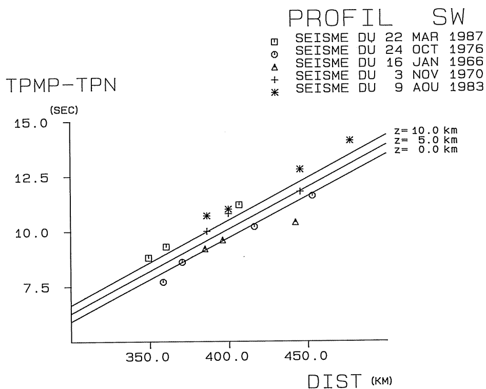
Fig. 17.- Différence de temps d'arrivées des phases PMP et Pn le long de deux profils à travers les stations du réseau LDG pour 5 séismes dans le Hainaut. Les valeurs théoriques obtenues pour un modèle crustal simple sont indiquées pour des profondeurs de foyers de 0, 5 et 10 km.
